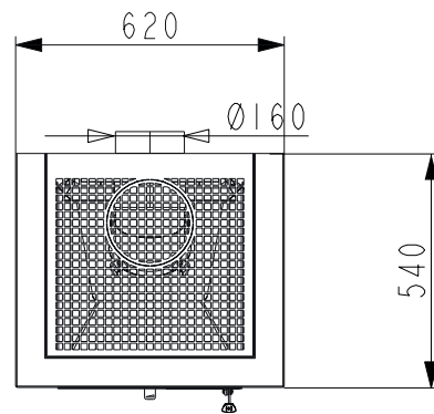
Rauchrohr-Anschluss wahlweise oben oder hinten
